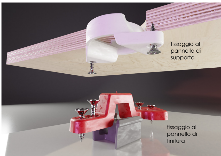
KIT L700903 con resistenza a trazione 8 kg (viti e spine non fornite con il kit)
